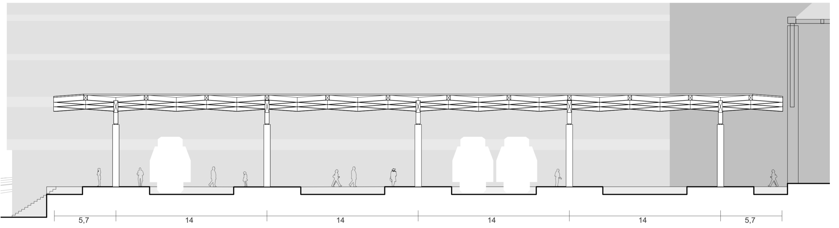
Section A-A 1-200
