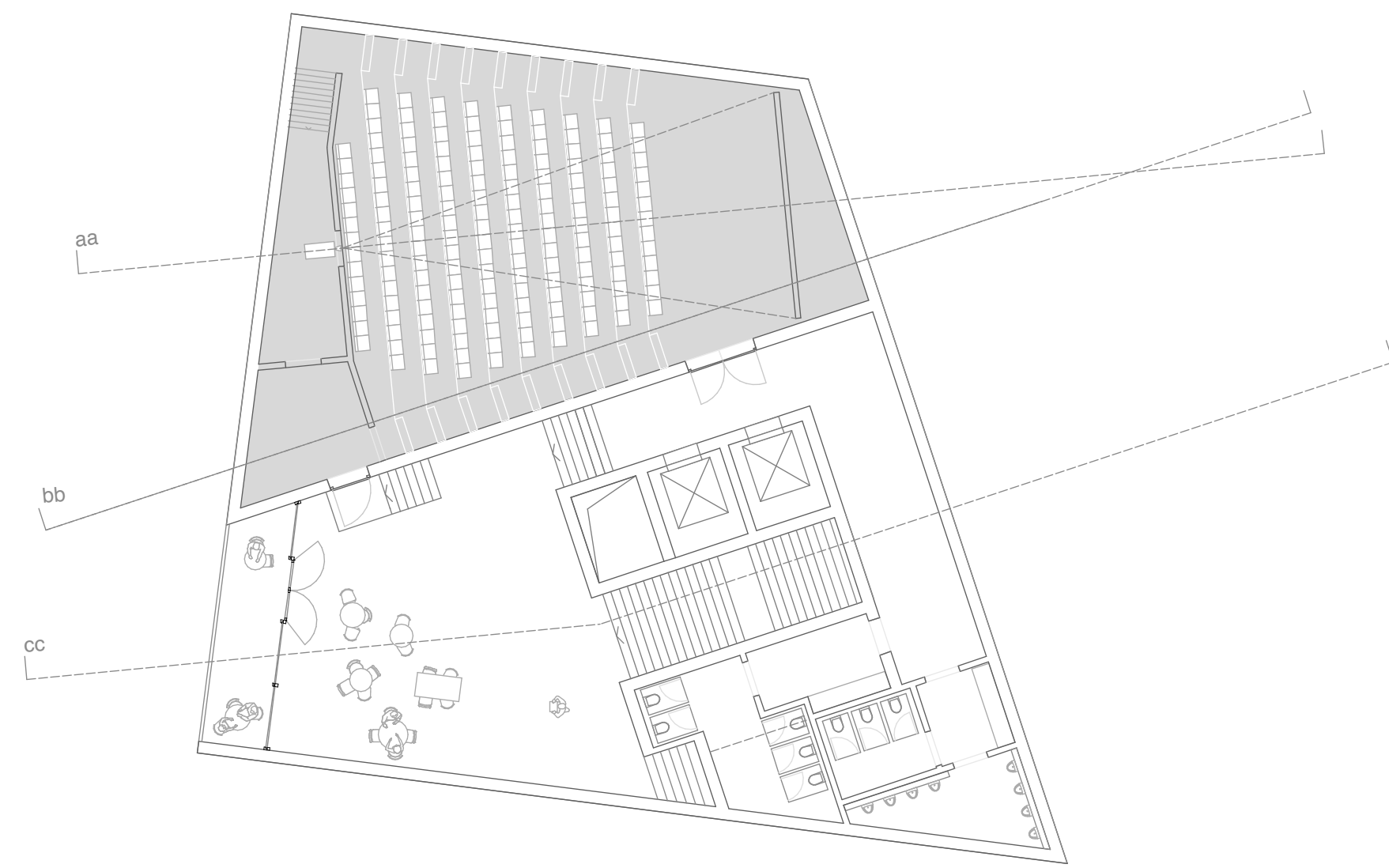
Grundriss 3.OG | 1:200
