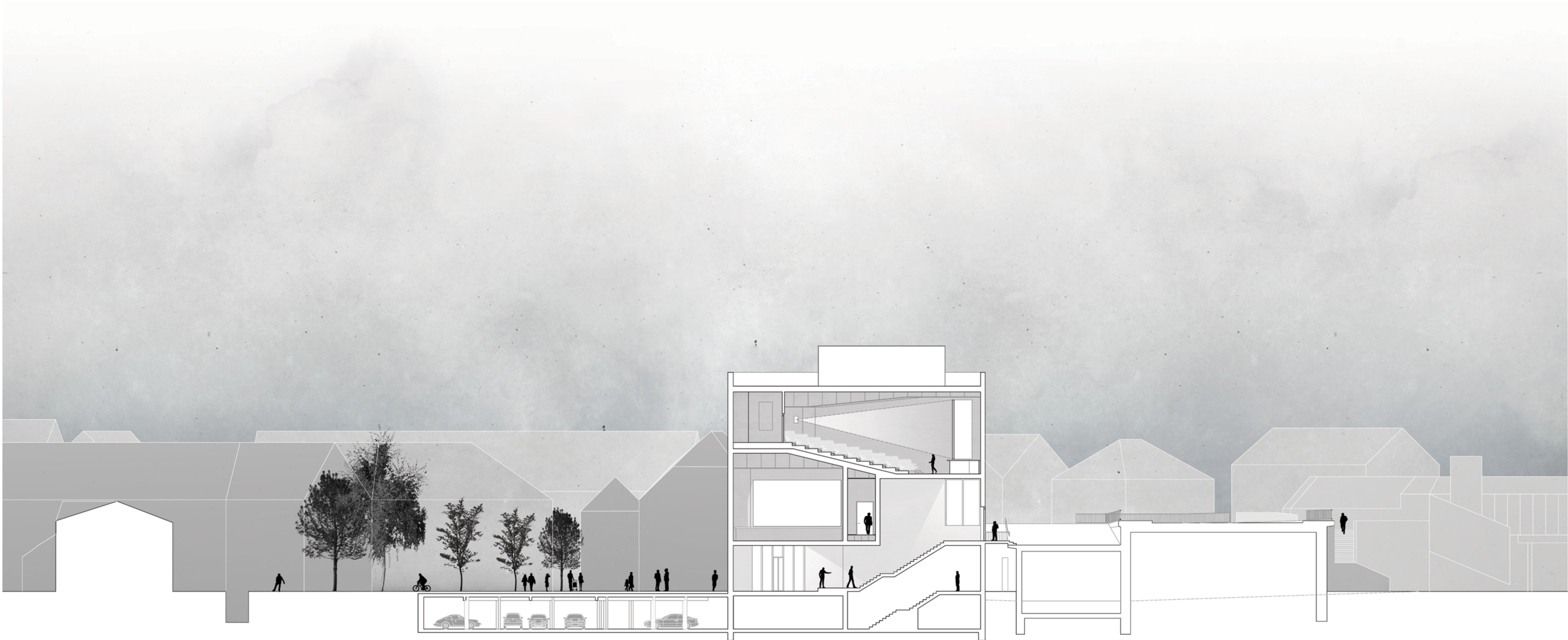
Schnitt bb | 1:200
