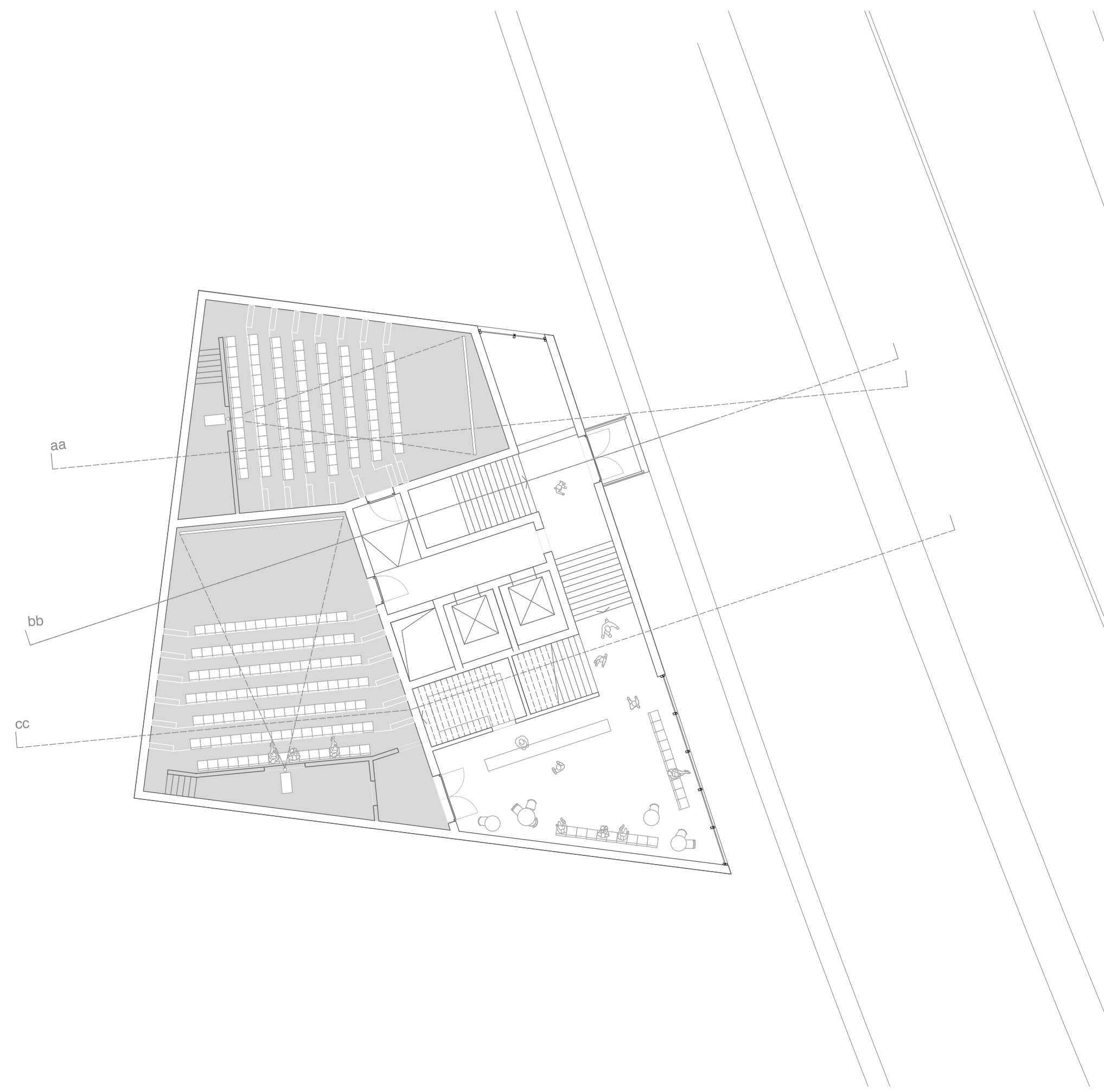
Grundriss 1.OG | 1:200
