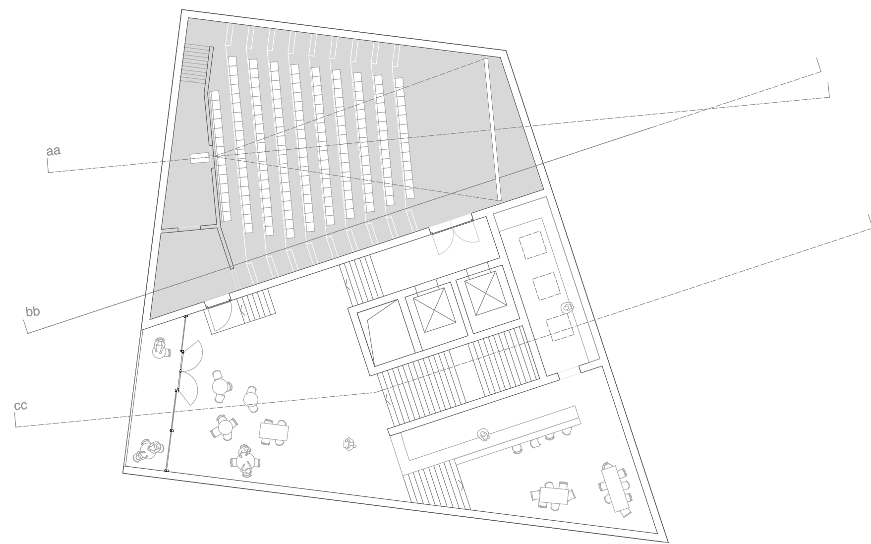
Grundriss 2.OG | 1:200
